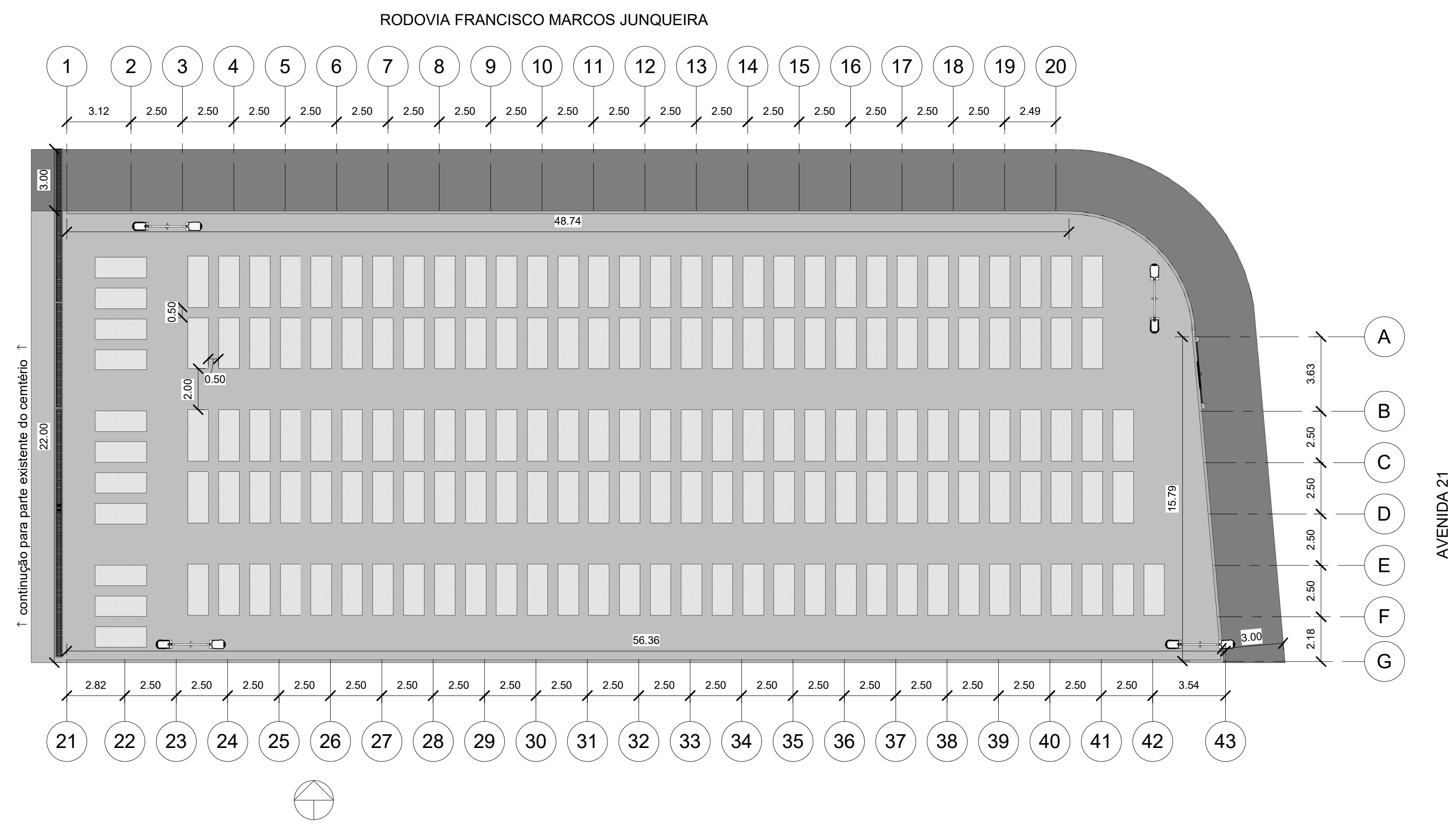
PLANTA BAIXA ESC: 1/150
