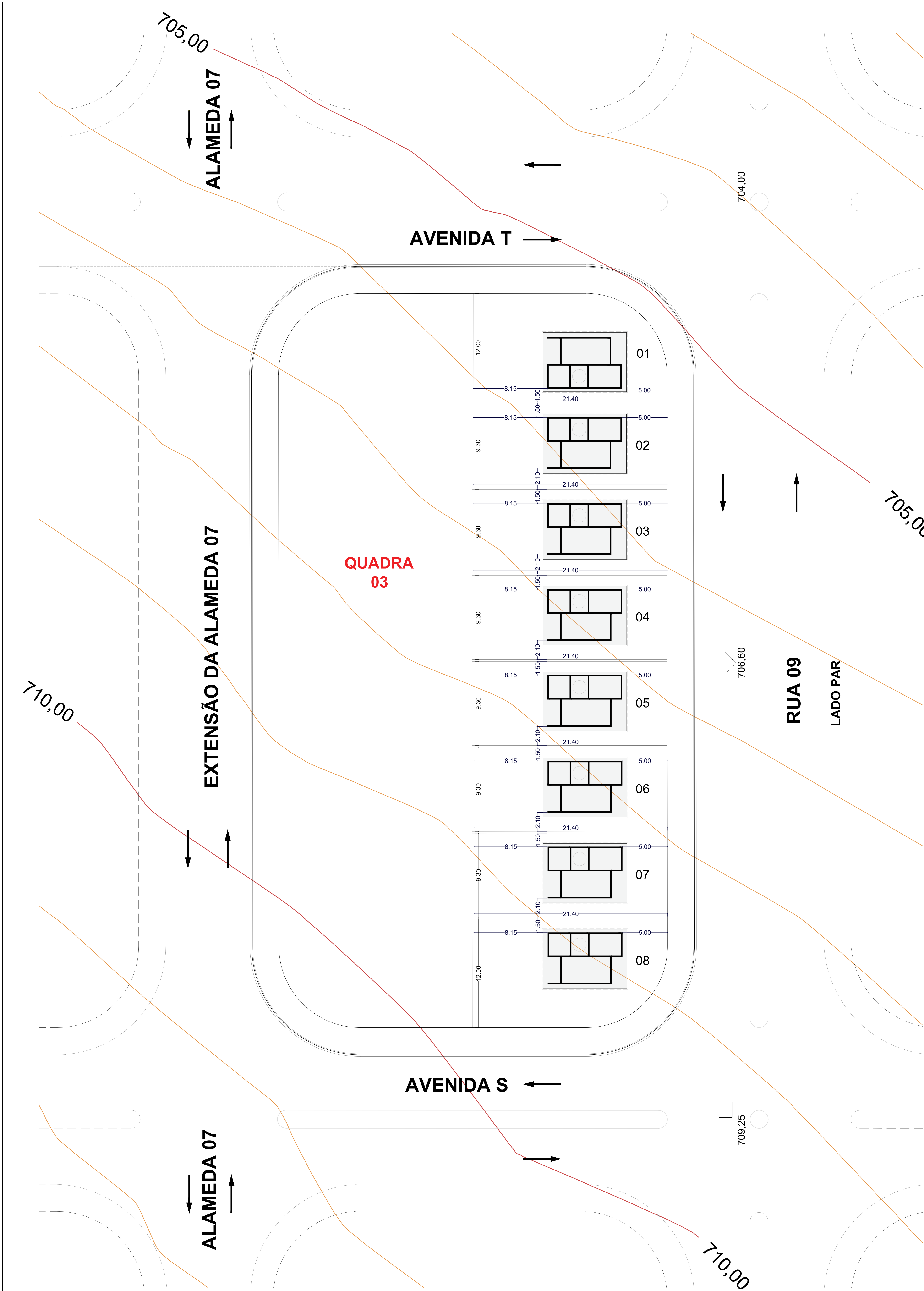
1. PLANTA DE LOCAÇÃO - UNIDADES HABITACIONAIS ESC: 1/200
