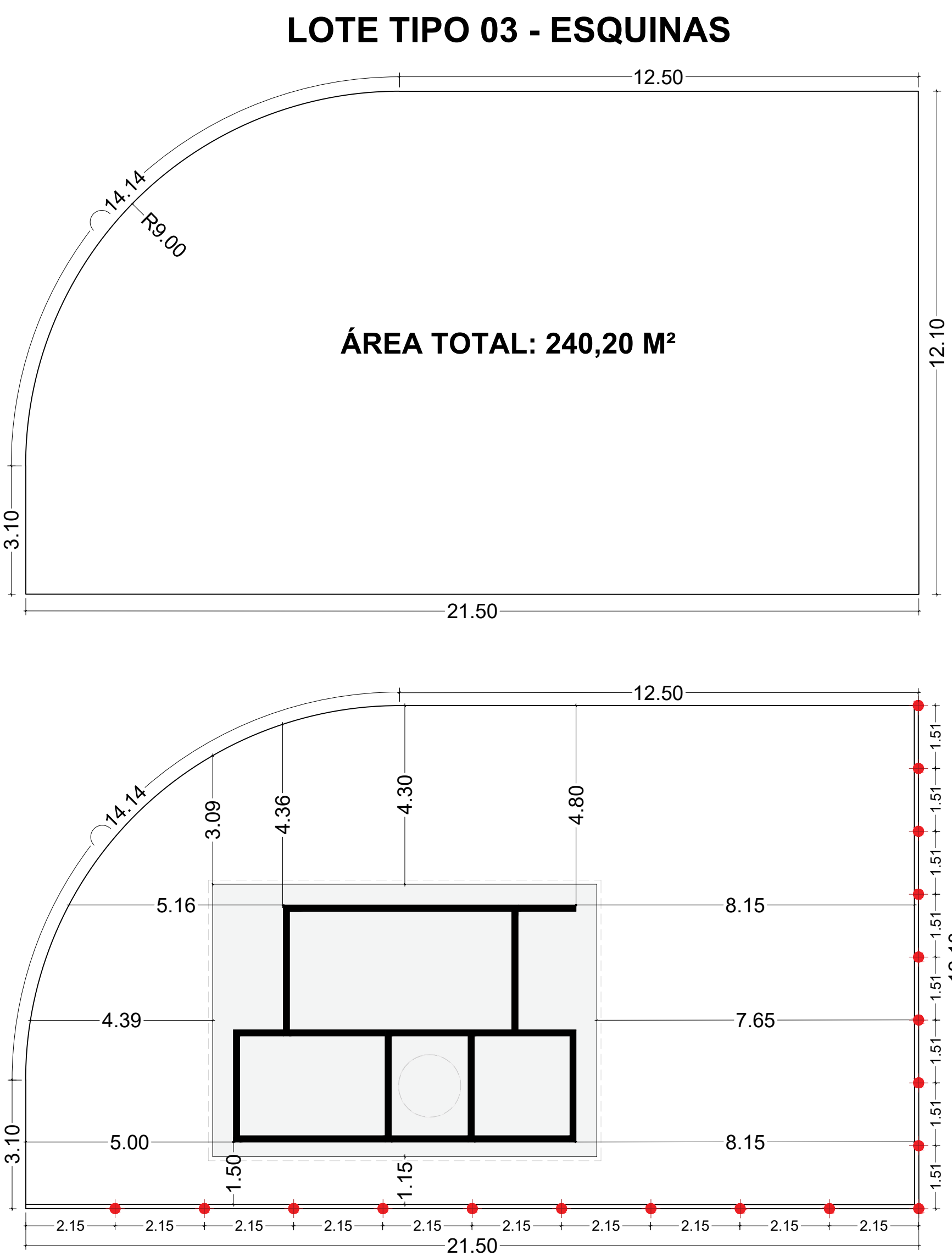
2. DETALHAMENTO DOS LOTES ESC: 1/100
