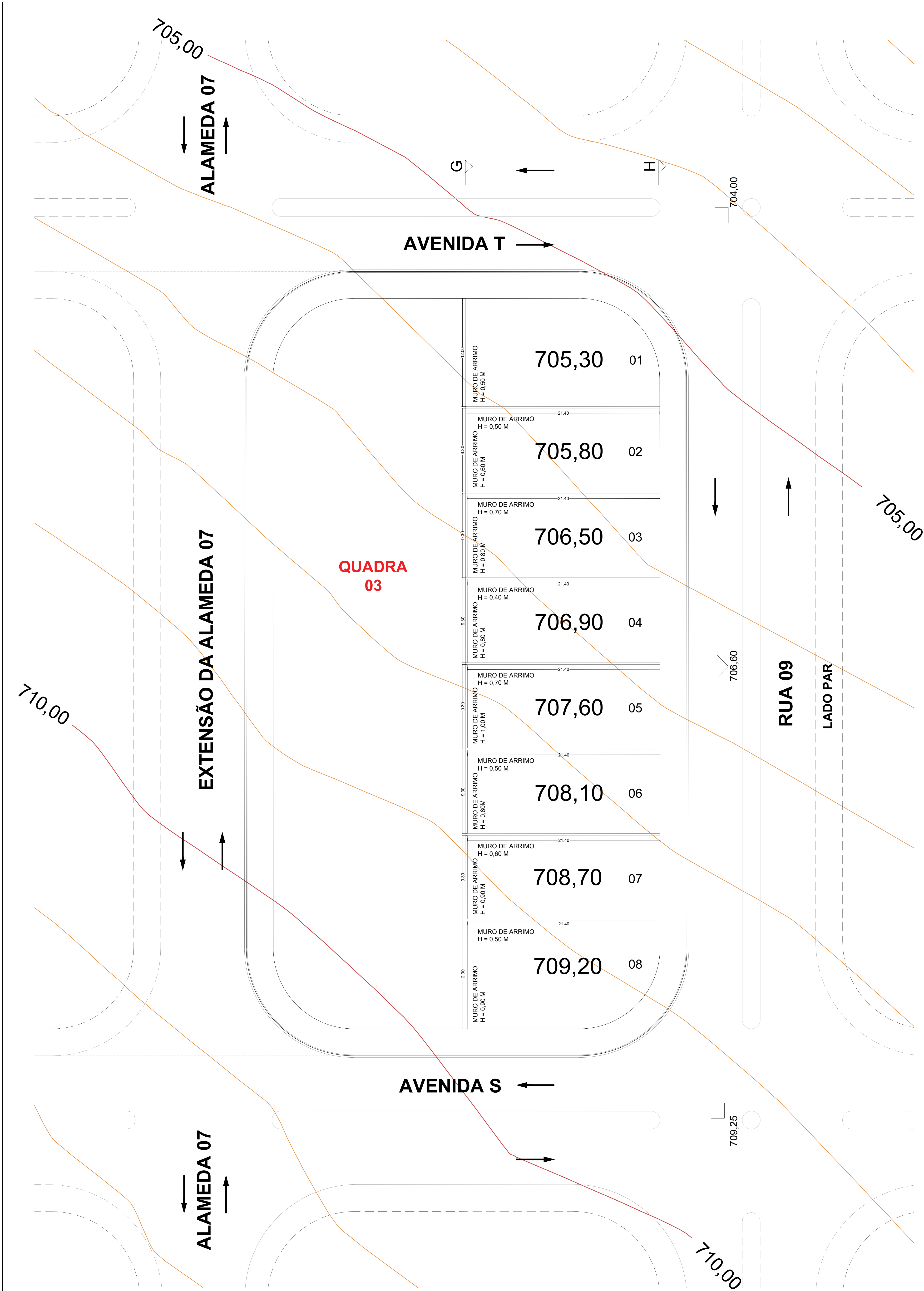
1. MARCAÇÃO DE COTAS DE NÍVEL ESC: 1/200
