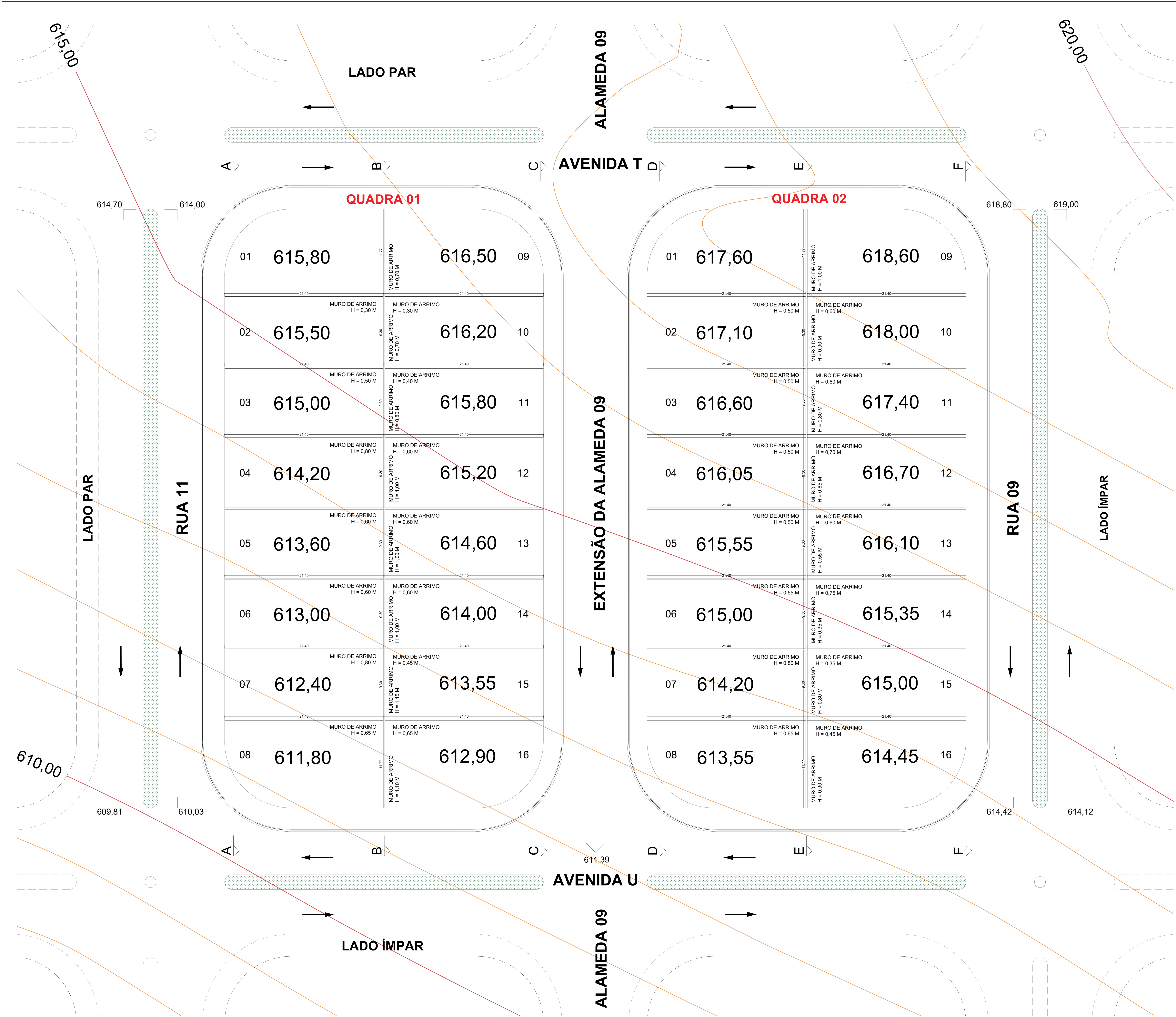
1. MARCAÇÃO DE COTAS DE NÍVEL ESC: 1/200
