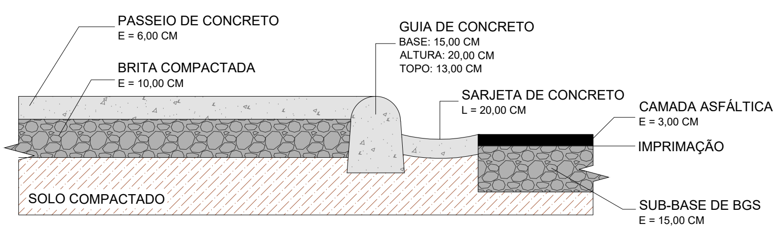
3. DETALHAMENTO DO PAVIMENTO ESC: 1/10
