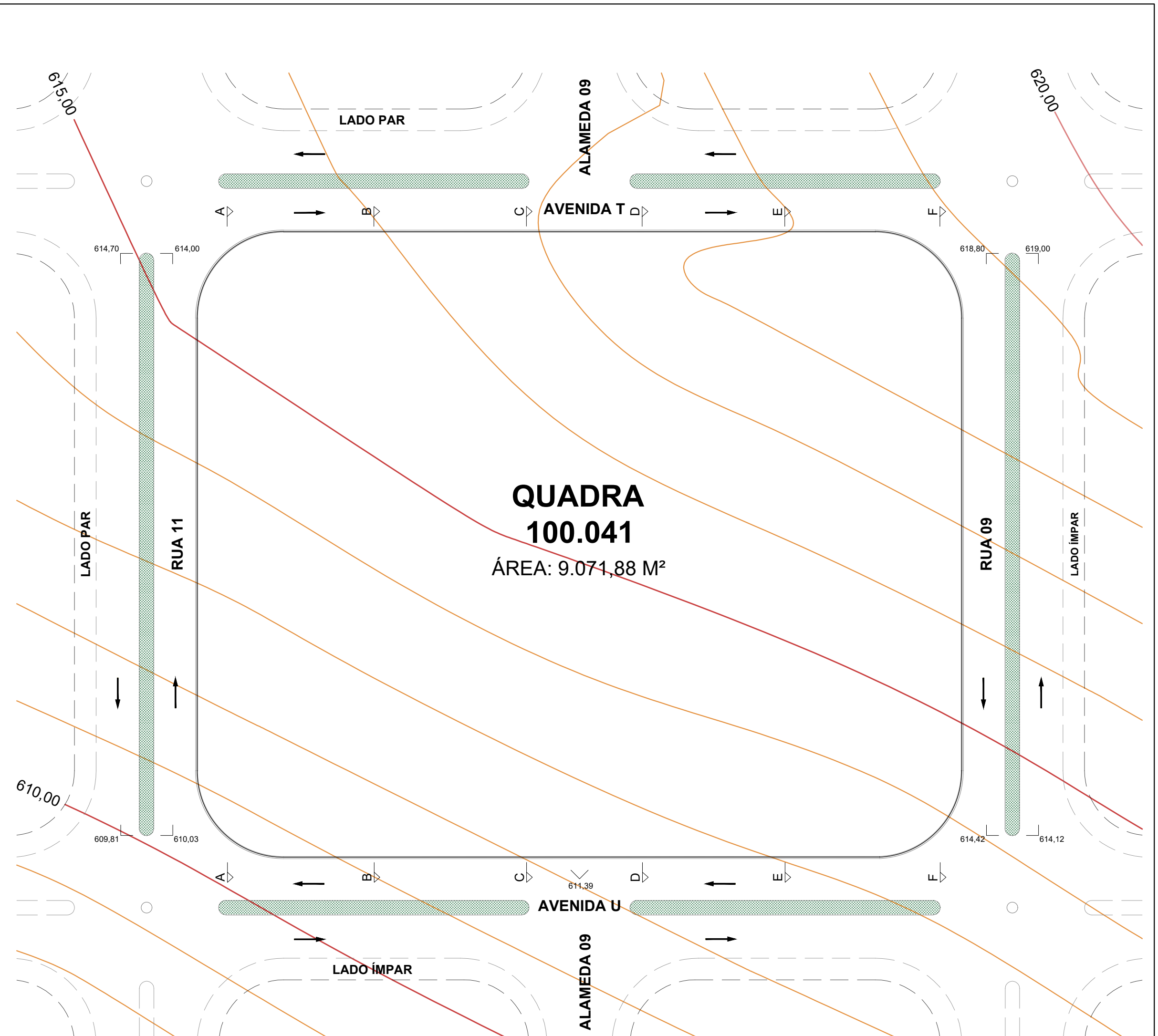
2. SITUAÇÃO DA QUADRA ESC: 1/500
