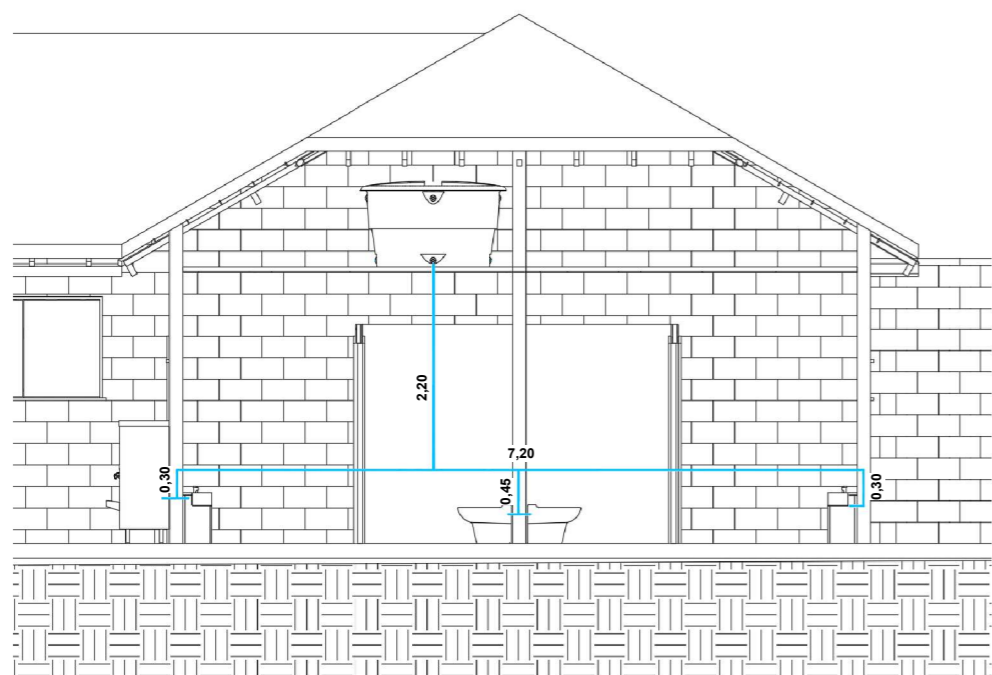
ABASTECIMENTO - CORTE 1
