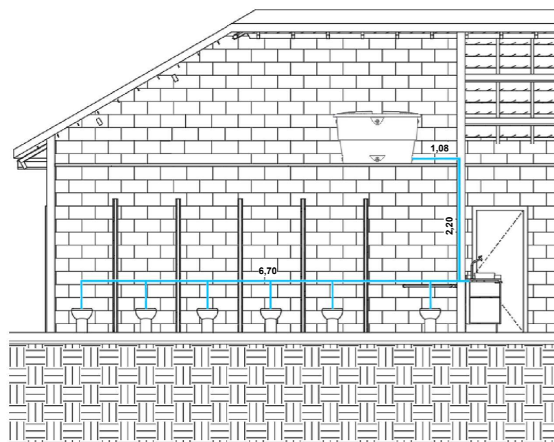
ABASTECIMENTO - CORTE 2
