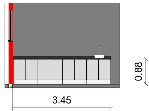
PIA SALA DOS PROFESSORES 1:50
