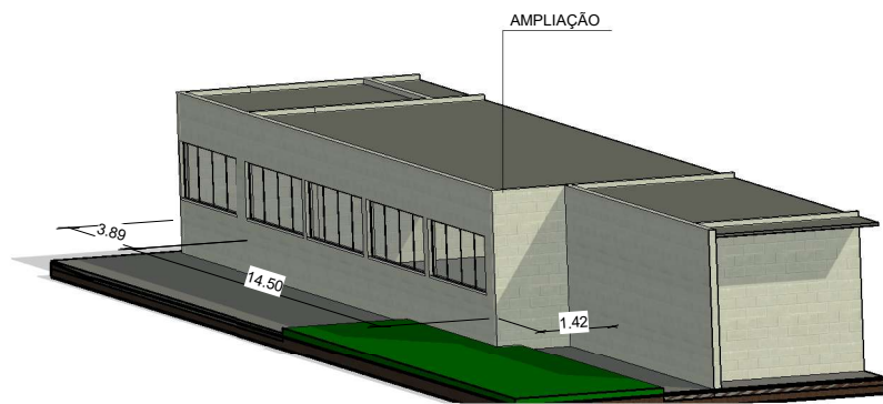
AMPLIAÇÃO REFEITÓRIO E DEPÓSITO 1:100
