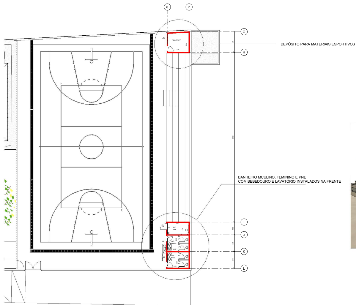
PLANTA BAIXA - QUADRA DE ESPORTES ESC. 1/75
