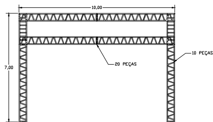
VISTA FRONTAL ESC: 1/100
