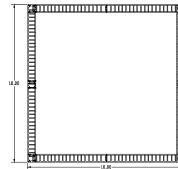
PLANTA BAIXA ESC: 1/100
