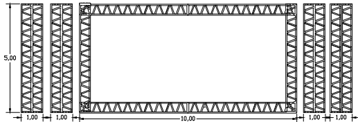
VISTA FRONTAL ESC: 1/100
