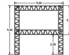
VISTA FRONTAL ESC: 1/100
