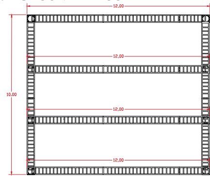
PLANTA BAIXA ESC: 1/100
