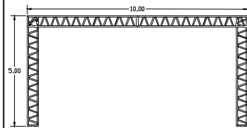
VISTA FRONTAL ESC: 1/100
