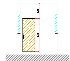
CORTI B-B ESC. 1/100
