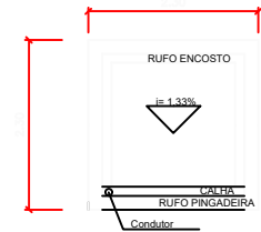
PLANTA DE COBERTURA ESC. 1/100
