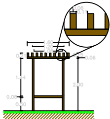
PERSPECTIVA BARRIL ESC 1/200
