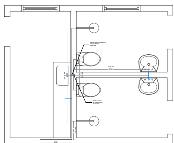
5. SISTEMA DE ABASTECIMENTO
