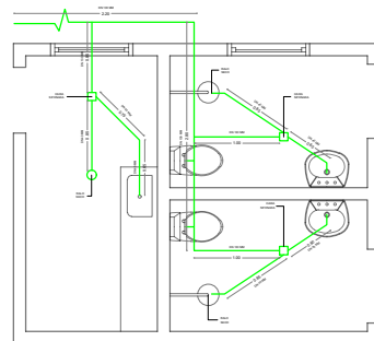
6. SISTEMA DE ESGOTAMENTO
