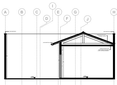
2. CORTE B-B
