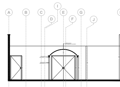
4. CORTE D-D
