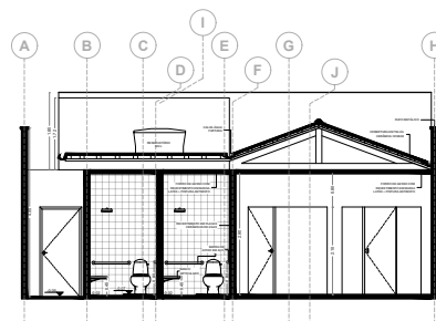
3. CORTE C-C
