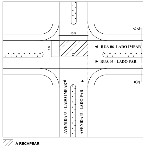
01. PLANTA DE SITUAÇÃO ESC: 1/1000
