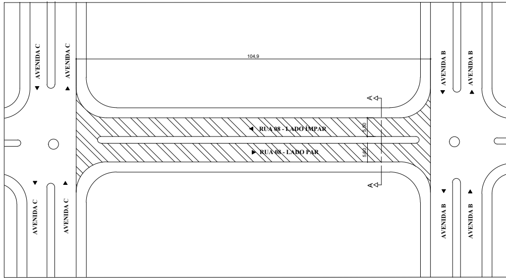
01. PLANTA DE SITUAÇÃO ESC: 1/1000
