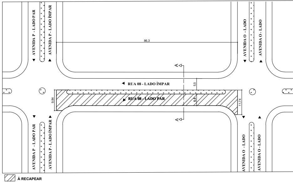
01. PLANTA DE SITUAÇÃO ESC: 1/1000
