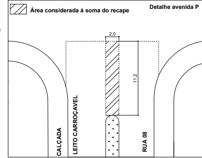
04. DETALHE DA EXTREMIDADE DO CANTEIRO ESC: 1/50
