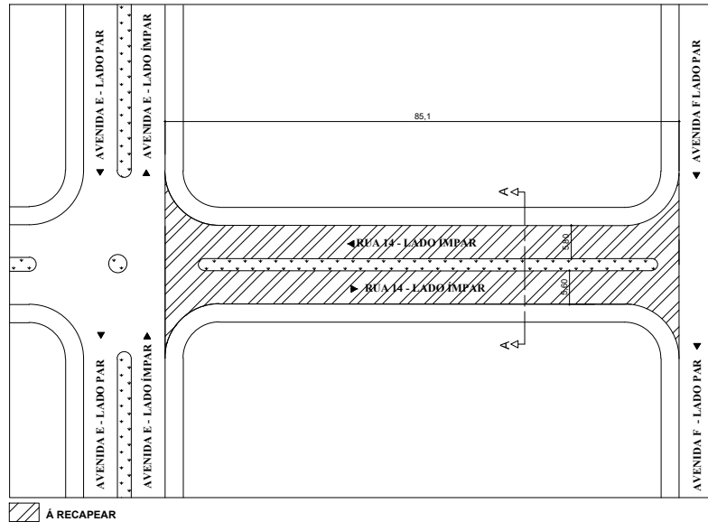
01. PLANTA DE SITUAÇÃO ESC: 1/1000
