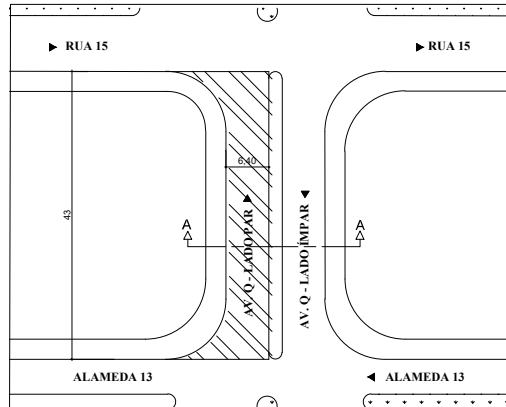
01. PLANTA DE SITUAÇÃO ESC: 1/1000
