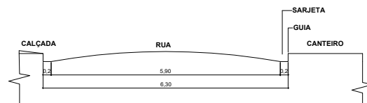
02. CORTE TRANSVERSAL A-A DAS RUAS ESC: 1/100
