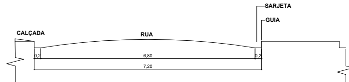
02. CORTE TRANSVERSAL A-A DAS RUAS ESC: 1/100
