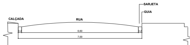
02. CORTE TRANSVERSAL A-A DAS RUAS ESC: 1/100
