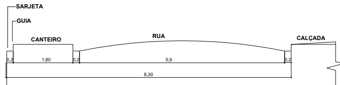
02. CORTE TRANSVERSAL A-A DAS RUAS ESC: 1/100
