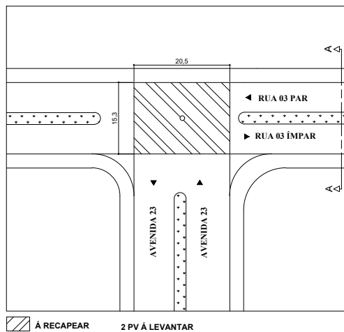
01. PLANTA DE SITUAÇÃO ESC: 1/1000
