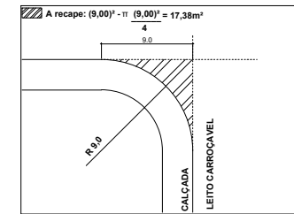
04. DETALHE DO RAIOS ESC: 1/10
