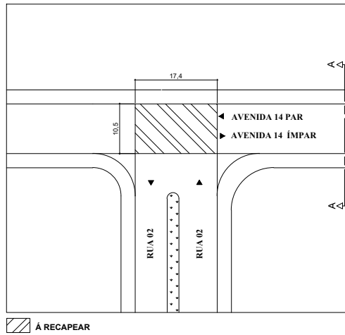
01. PLANTA DE SITUAÇÃO ESC: 1/1000
