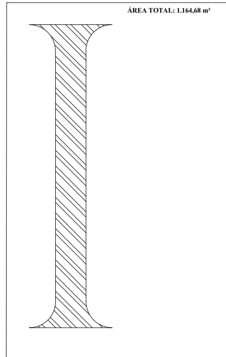
03. ÁREA A SER RECAPEADA ESC: 1/1000
