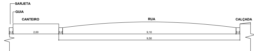
03. CORTE TRANSVERSAL A-A DAS RUAS ESC: 1/100
