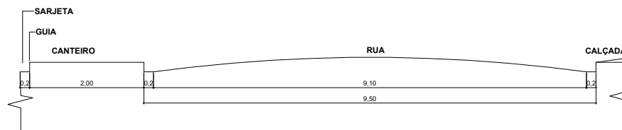
03. CORTE TRANSVERSAL A-A DAS RUAS ESC: 1/100
