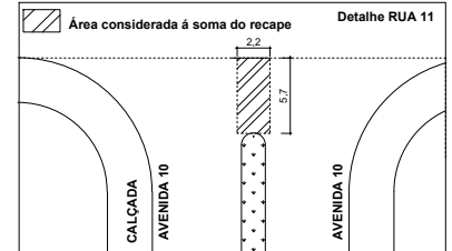
06. DETALHE DA EXTREMIDADE DO CANTEIRO ESC: 1/50
