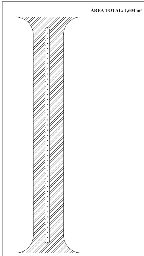
03. ÁREA A SER RECAPEADA ESC: 1/1000
