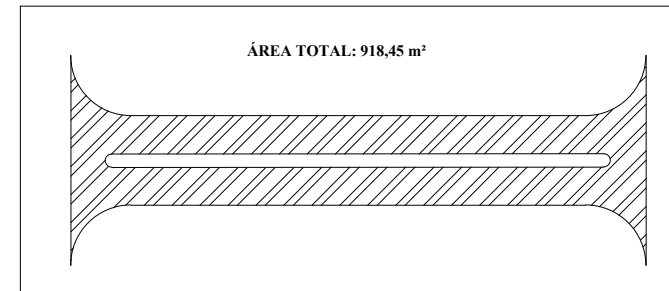
06. ÁREA A SER RECAPEADA ESC: 1/1000
