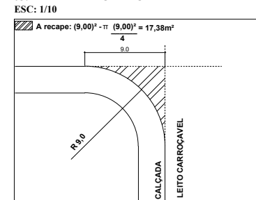
03. DETALHE DO RAIO ESC: 1/10
