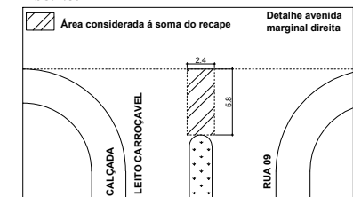
04. DETALHE DA EXTREMIDADE DO CANTEIRO ESC: 1/50
