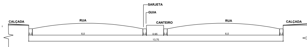
02. CORTE TRANSVERSAL A-A DAS RUAS ESC: 1/100
