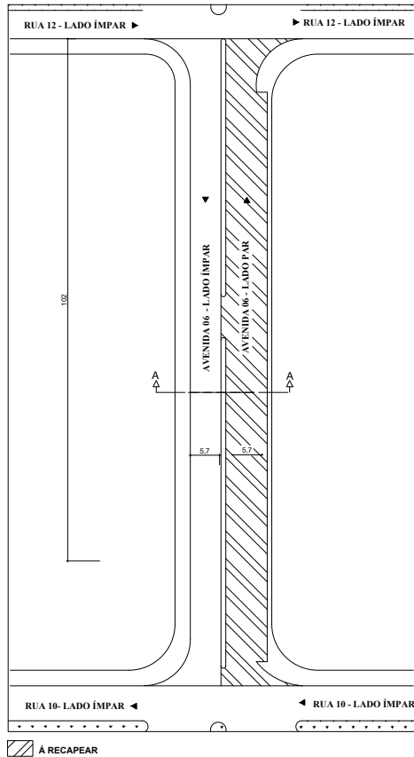
01. PLANTA DE SITUAÇÃO ESC: 1/1000
