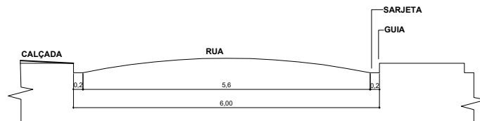
02. CORTE TRANSVERSAL A-A DAS RUAS ESC: 1/100
