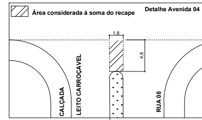
04. DETALHE DA EXTREMIDADE DO CANTEIRO ESC: 1/50
