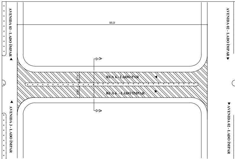
01. PLANTA DE SITUAÇÃO ESC: 1/1000
