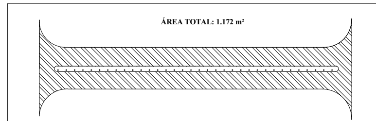
06. ÁREA A SER RECAPEADA ESC: 1/1000
