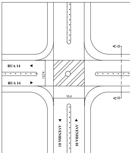
01. PLANTA DE SITUAÇÃO ESC: 1/1000
