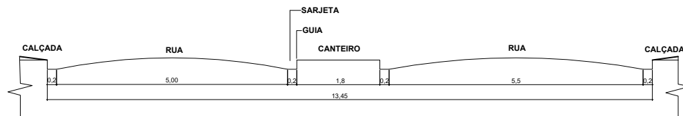
02. CORTE TRANSVERSAL A-A DAS RUAS ESC: 1/100
