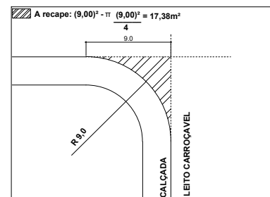
04. DETALHE DA EXTREMIDADE DO CANTEIRO
