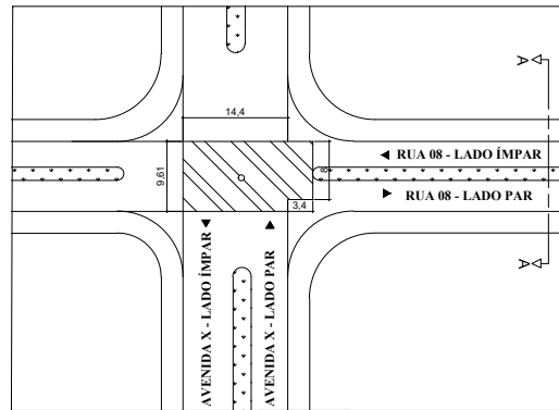
01. PLANTA DE SITUAÇÃO ESC: 1/1000
