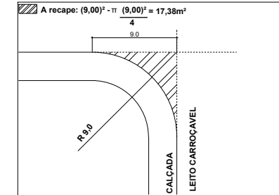
04. DETALHE DO RAIO ESC: 1/10
