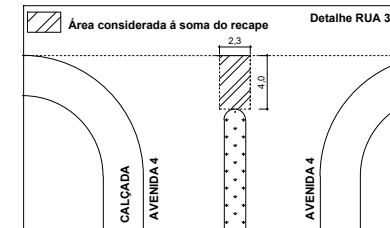
06. DETALHE DA EXTREMIDADE DO CANTEIRO ESC: 1/50
