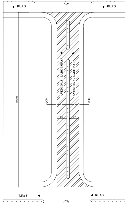
01. PLANTA DE SITUAÇÃO ESC: 1/1000
