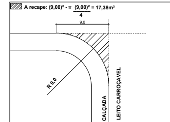
04. DETALHE DO RAIO RUA 01 ESC: 1/10
