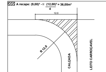
05. DETALHE DO RAIO RUA 03 ESC: 1/10
