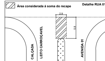
06. DETALHE DA EXTREMIDADE DO CANTEIRO ESC: 1/50
