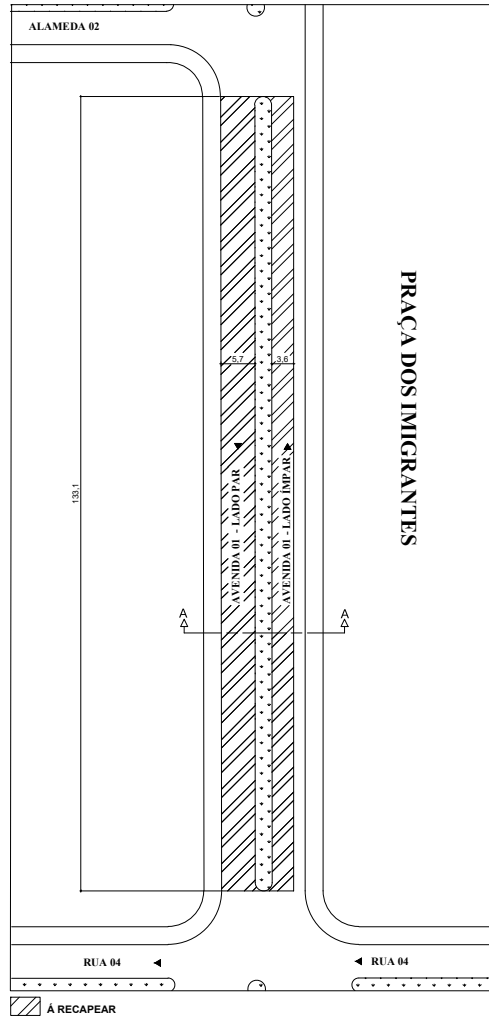
01. PLANTA DE SITUAÇÃO ESC: 1/1000
