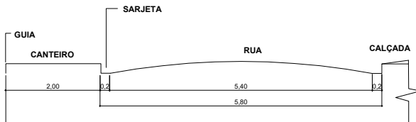
02. CORTE TRANSVERSAL A-A DAS RUAS ESC: 1/100
