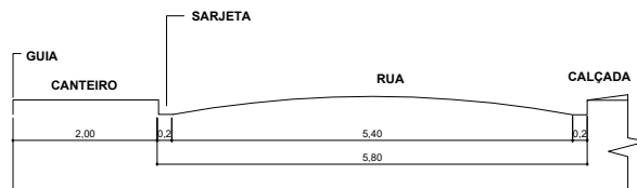
02. CORTE TRANSVERSAL A-A DAS RUAS ESC: 1/100
