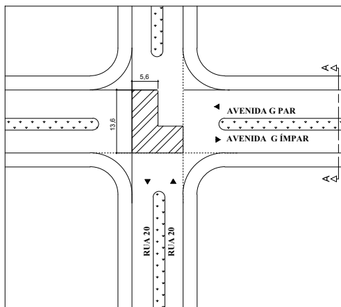
01. PLANTA DE SITUAÇÃO ESC: 1/1000
