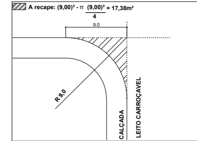
05. DETALHE DA EXTREMIDADE DO CANTEIRO ESC: 1/20
