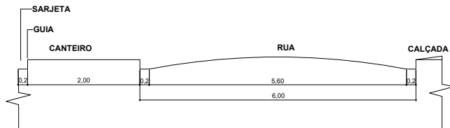
02. CORTE TRANSVERSAL A-A DAS RUAS ESC: 1/100
