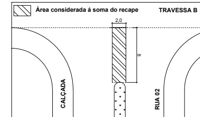
05. DETALHE DA EXTREMIDADE DO CANTEIRO ESC: 1/20
