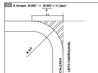
04. DETALHE DO RAIO ESC: 1/10
